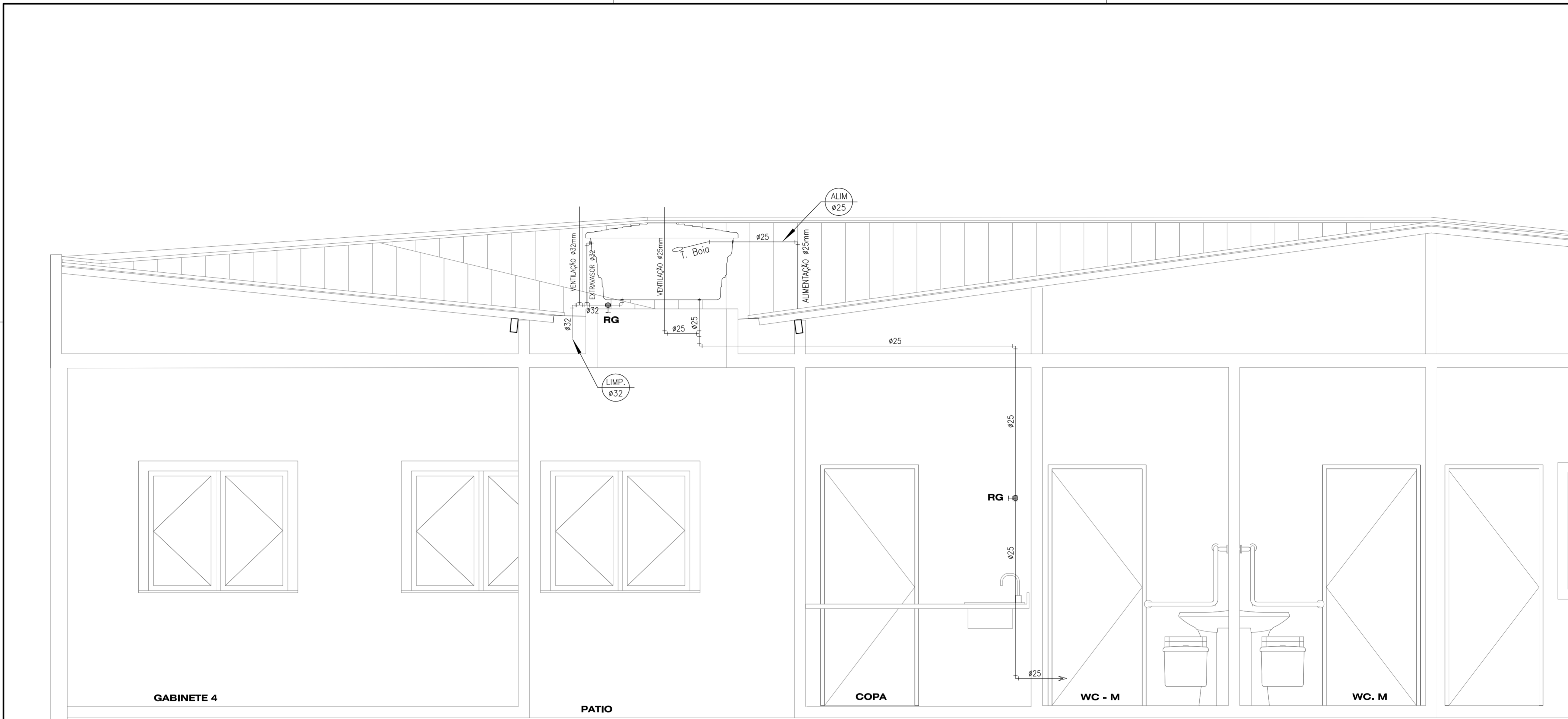
PERFIL DO BARRILETE ESC. 1/25
